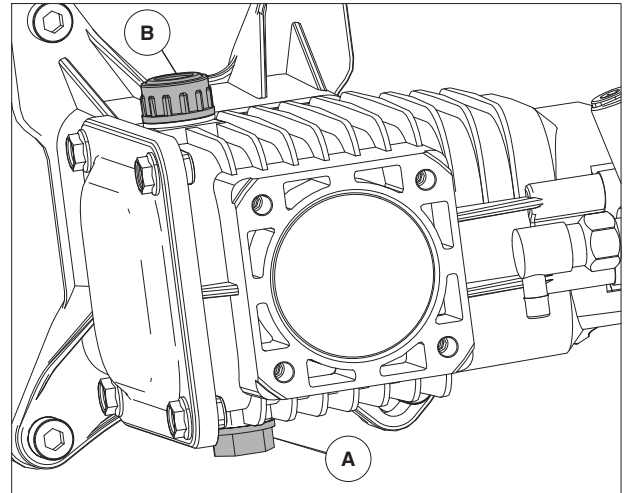
Figura 8 – Compruebe el aceite de la bomba
